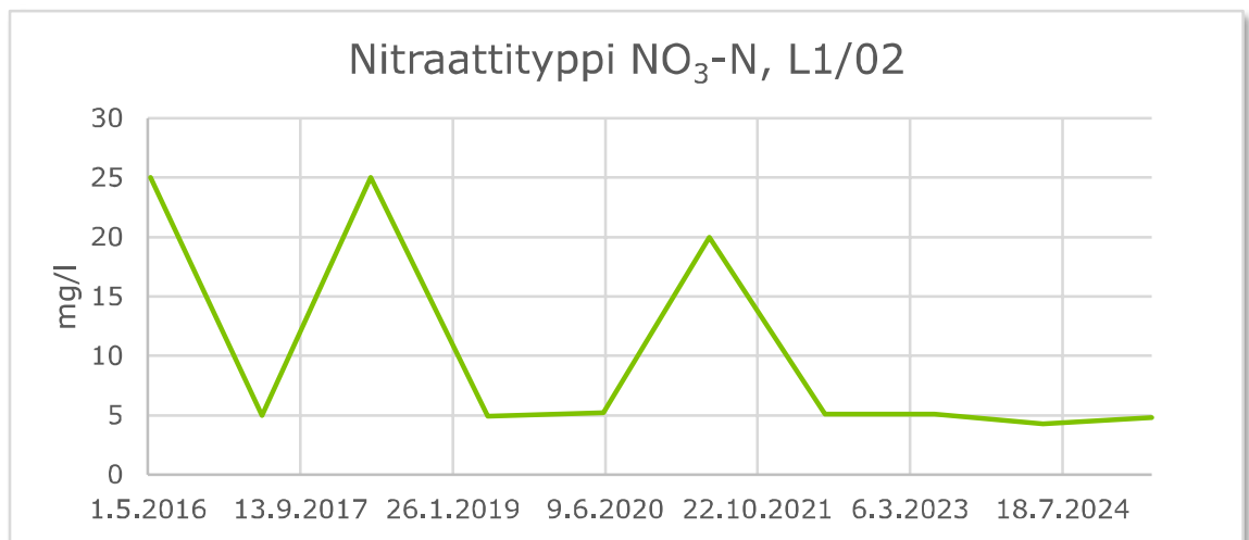
Kuva 6-7. Nitraattityypin pitoisuuden kehitys havaintoputkessa L1/02 vuosina 2016–2024.
