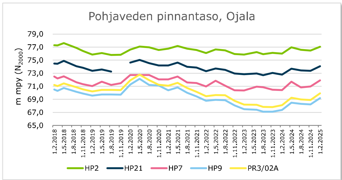
Kuva 6-3. Pohjaveden pinnantas tarkkailuun kuuluvista havaintoputkista 2018–2025.
